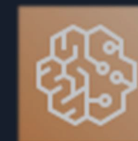
Amazon SageMaker
